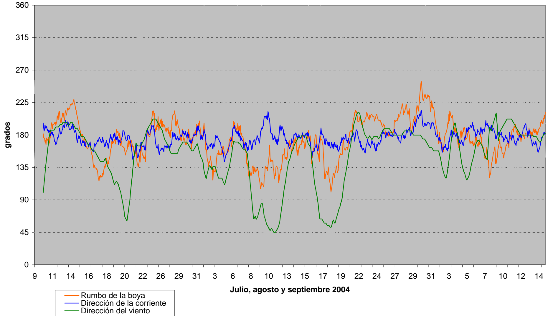
Tendencia media móvil de la dirección de la boya 42859, corriente y viento
