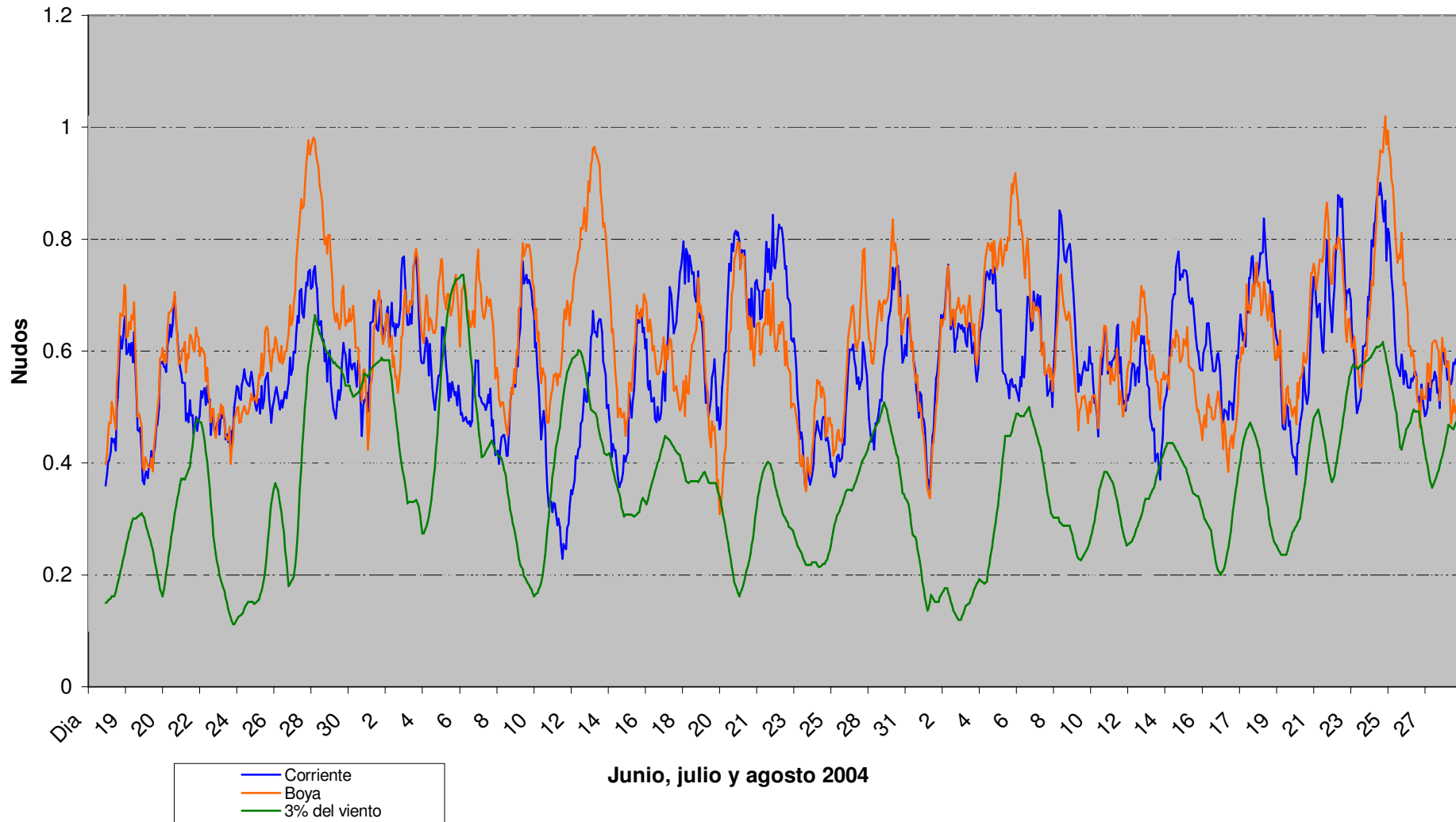
Tendencia media móvil de las velocidades (boya 42857)
