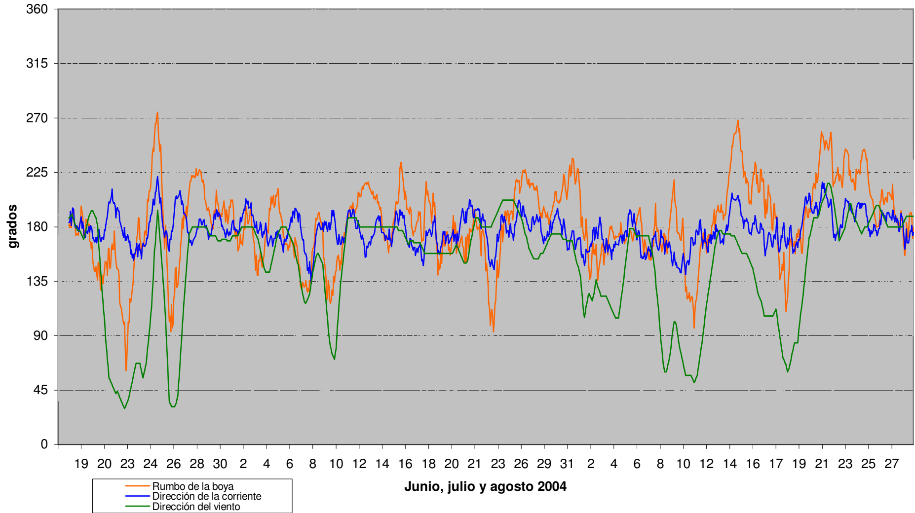
Tendencia media móvil de la dirección de la boya 42857, corriente y viento
