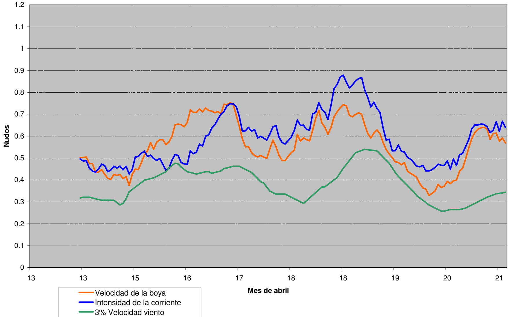
Tendencia media móvil de las velocidades de la boya, viento y corriente (Boya 42853)
